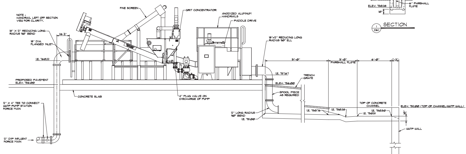
SECTION A-A
