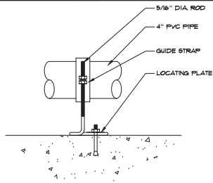
PIPE SUPPORT SCALE: N.T.S.
