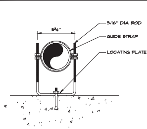
PIPE SUPPORT SCALE: N.T.S.
