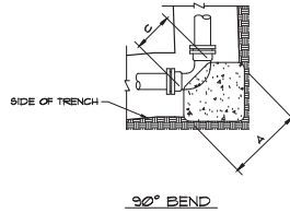
90° BEND
