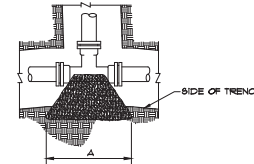
TEE
